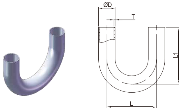
DT-4.1.1-7 180° WELD ELBOW (DT-23)
