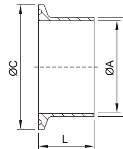
3A-1.0"~12" SMS-DN25~DN100 DIN-DN10~DN100 DIN(ISO)-DN15~DN200
