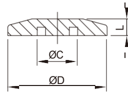
Blank Flange
