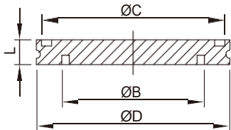
Blank Flange
